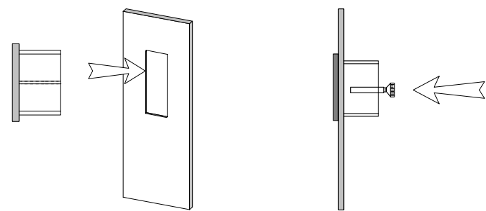
主体部分安装
