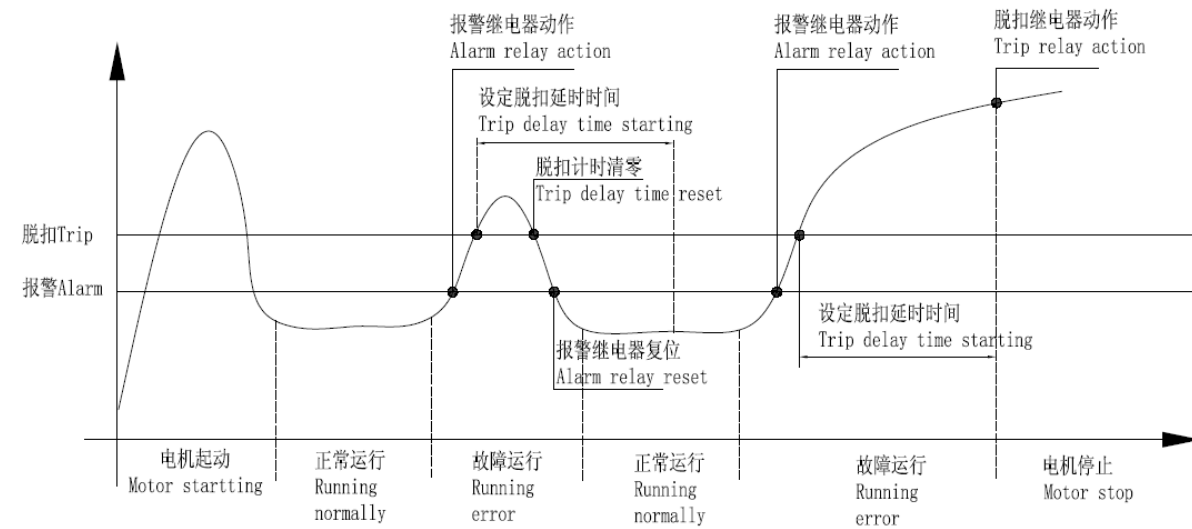
保护器动作示意图 Schematic diagram
