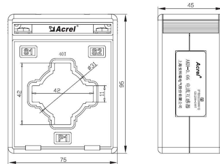
互感器部分 (0.1A~100A)
