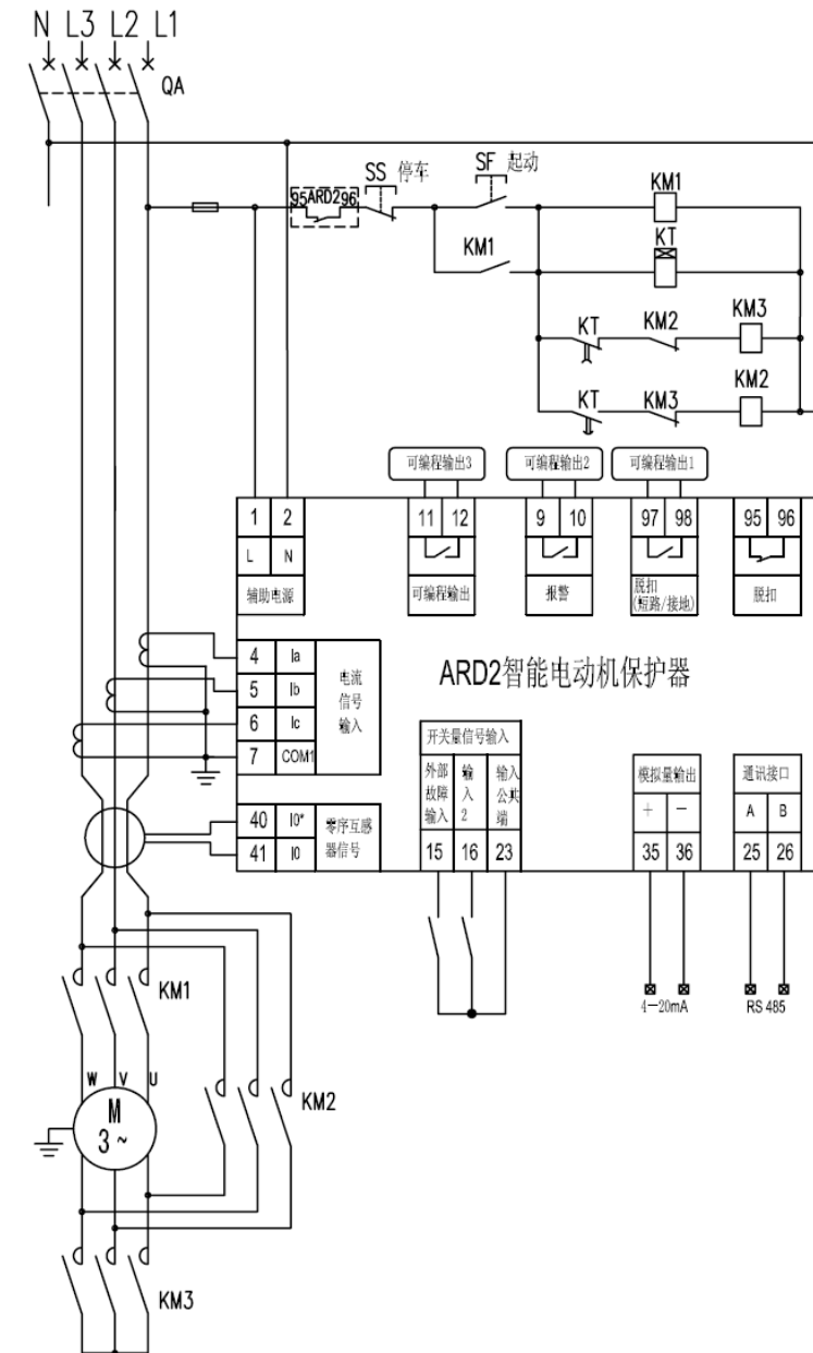
ARD2 电动机保护器 Y-△ 起动模式接线图
