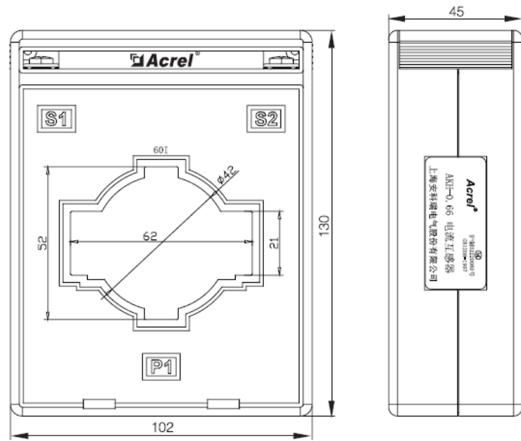
互感器部分 (250A~800A)
